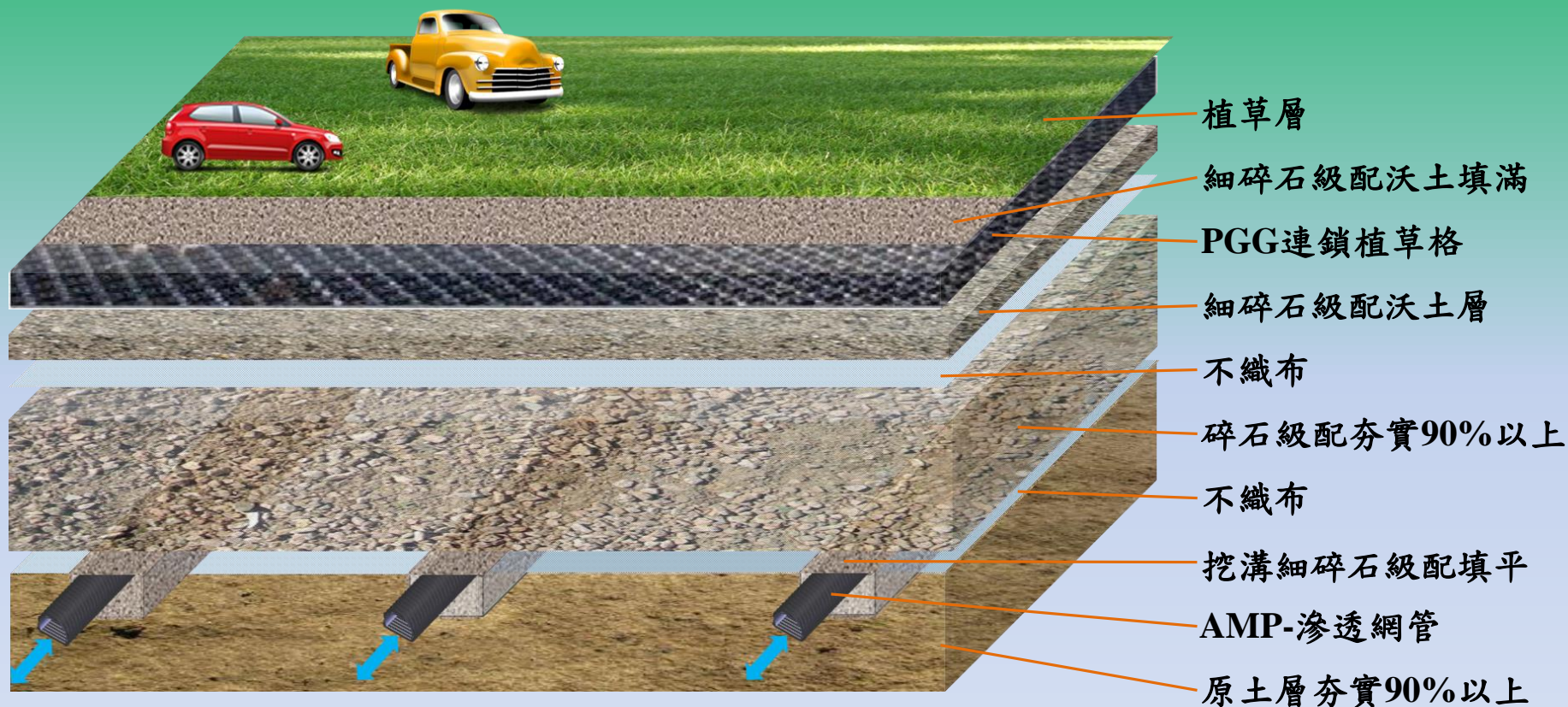
PGG植草格鋪面灌溉排水停車場、車道施工步驟 示意圖
